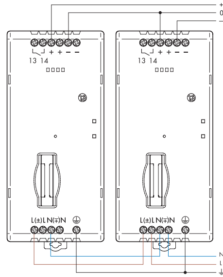
Последовательное подключение
