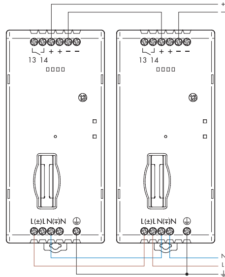
Последовательное подключение
