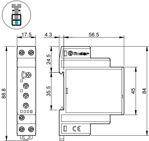
Тип 70.41 Винтовой клеммы
