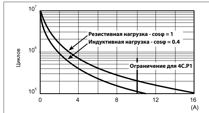
F 4С - Электрическая долговечность (АС) при ном. нагрузке, Типы 4С.01/Р1
