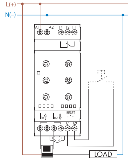
70.51 с подключением ТА
