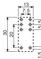
95.15.2 Вид сбоку
