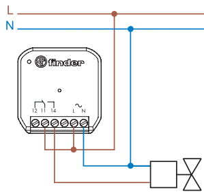
2-проводное
