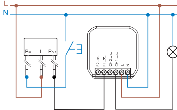
Примеры приложений с реле 13.22
