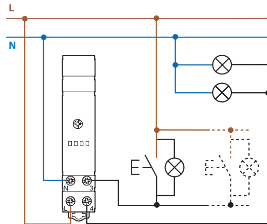
4-проводное соединение
