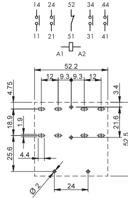
Вид со стороны выводов
