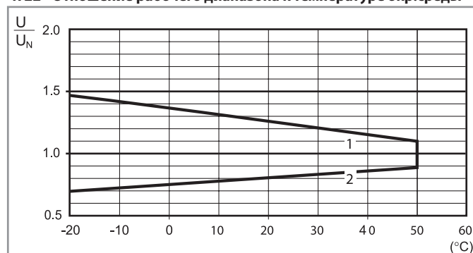
R 22 - Отношение рабочего диапазона к температуре окр.среды
