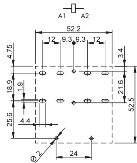
Вид со стороны выводов
