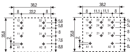
62.22 Вид со стороны выводов
