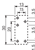
95.13.2 Вид сбоку
