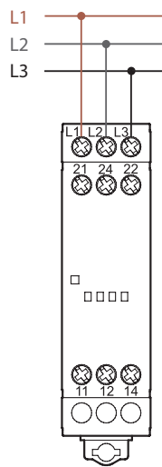
Тип 70.51 и 70.51 NFC
