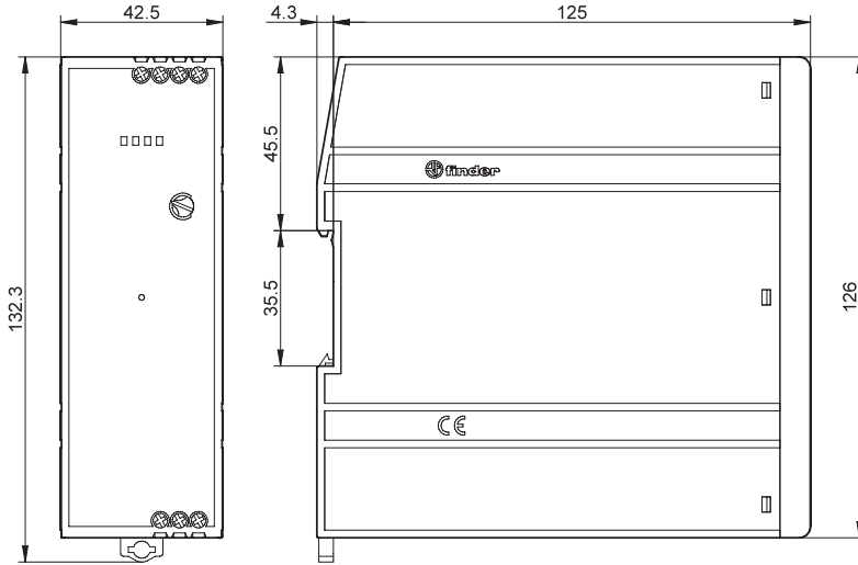
Тип 78.2А Винтовой клеммы
