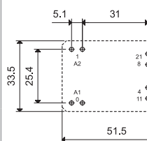
Вид со стороны выводов
