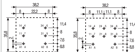
62.22 - 4300 Вид со стороны выводов
