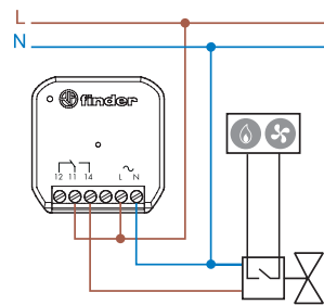
4-проводное
