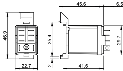
056.27 con relé
