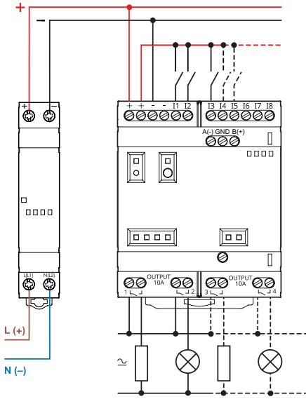
78.1B - Conexión de la fuente de alimentación
