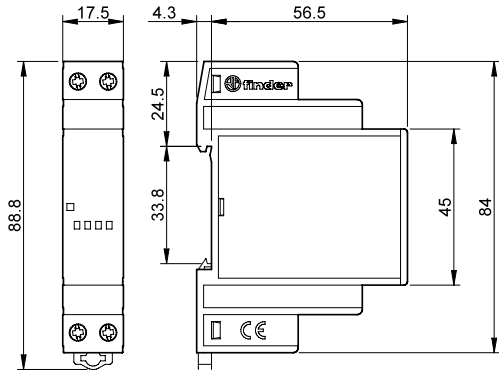
Tipo 78.36 / 78.50 / 78.60 Borne de jaula
