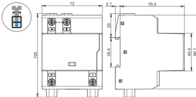
Tipo 7P.13.9.000.x006 Borne de jaula
