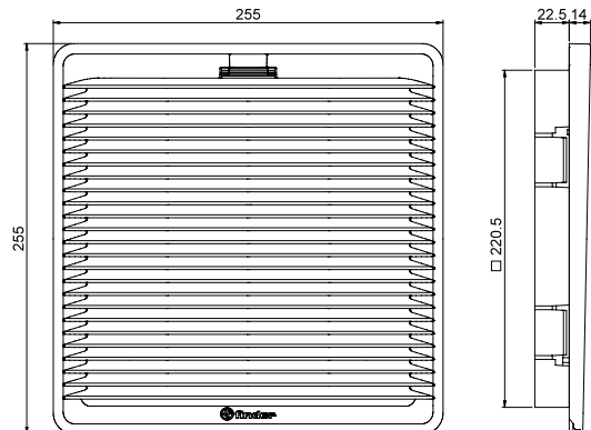
Tipo 7F.0x.0.000.4000
