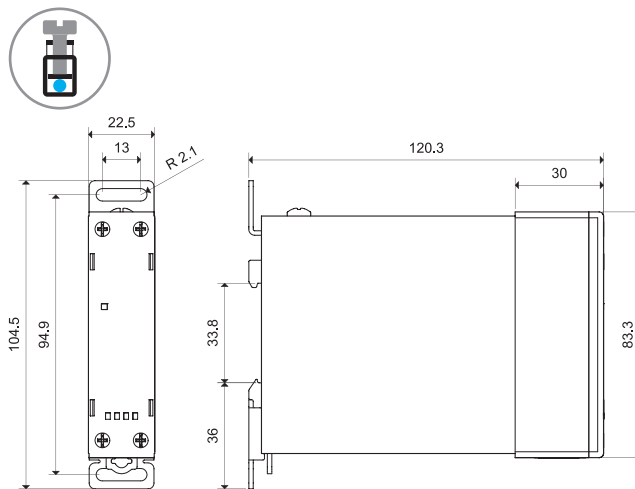
Tipo 77.x5
