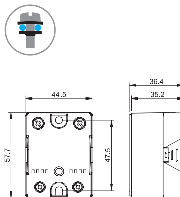
Tipo 77.x5
