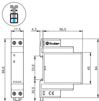
Tipo 77.01 DC
