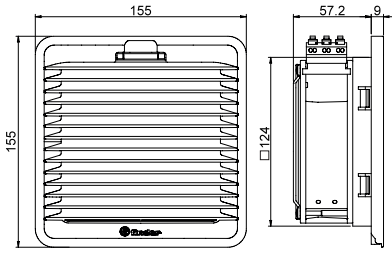
Tipo 7F.xx.x.xxx.2055
