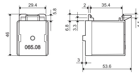
065.08
