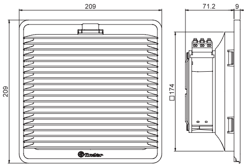
Tipo 7F.xx.x.xxx.3100
