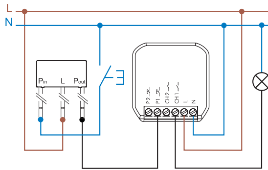
Ejemplo de aplicación con tipo 13.22
