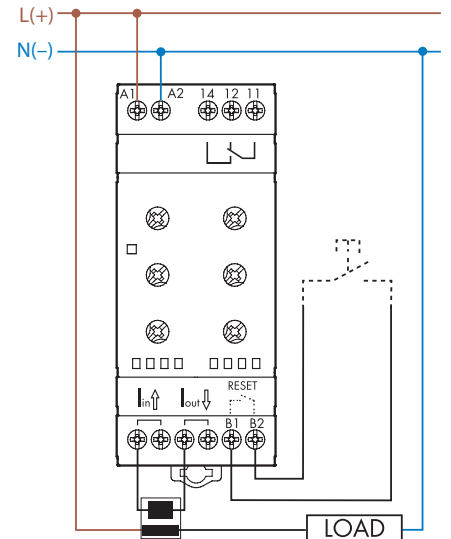
70.51 con conexión TA
