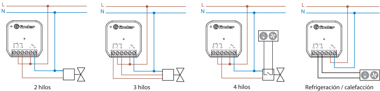
Tipo 13.21.8.230.S000 Electroválvula de 2, 3 y 4 hilos o conexión directa
