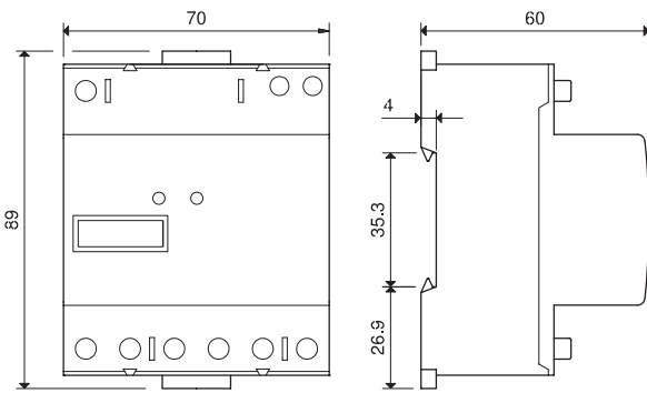
Tipo 7E.36.8.400.0010
