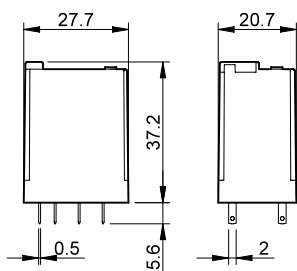
Tipo 55.32
