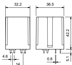
Tipo 65.61
