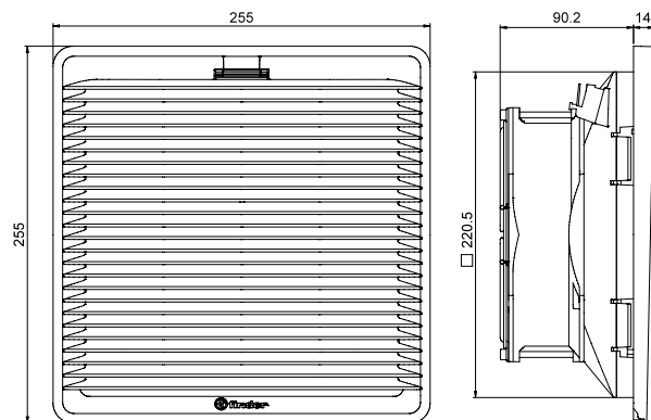
Tipo 7F.xx.x.xxx.4250
