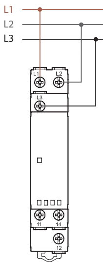
Tipo 70.61
