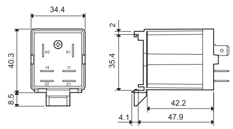
065.07 con relé
