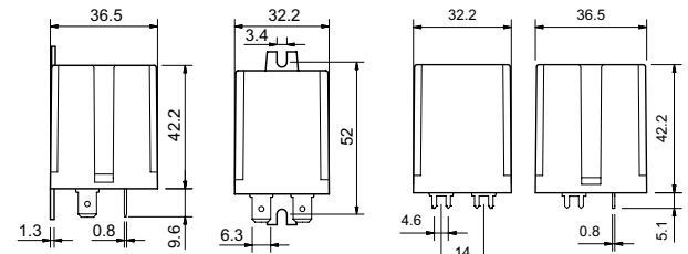
Tipo 65.31- 4300
