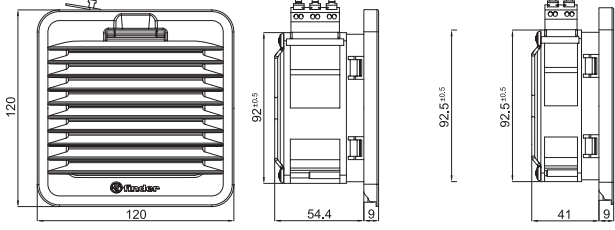
Tipo 7F.xx.x.xxx.1020
