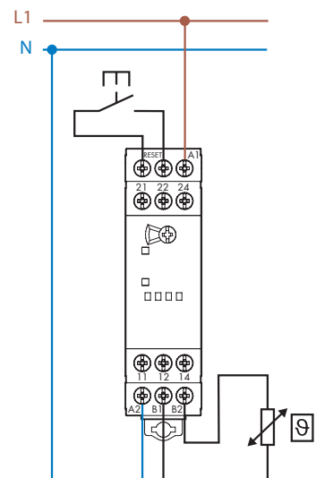
Tipo 70.92
