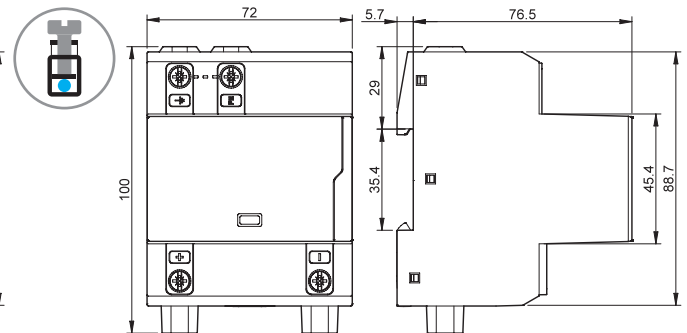
Tipo 7P.13.9.500.x006 Borne de jaula
