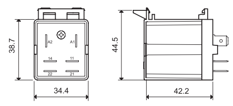
065.08 con relé
