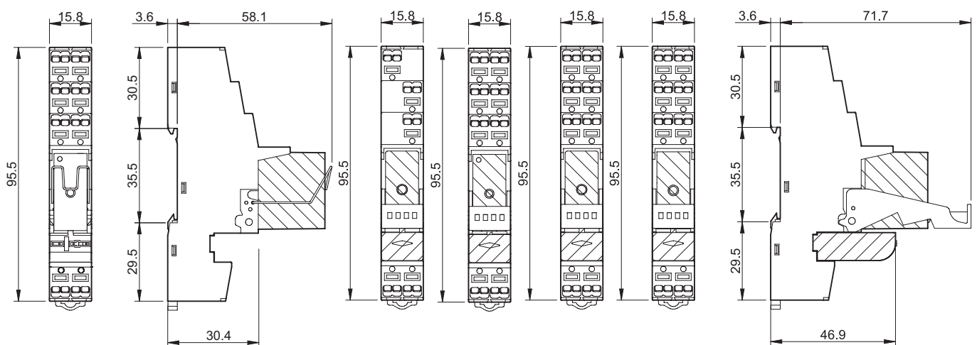
Tipo 48.P2
