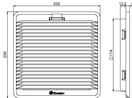
Tipo 7F.0x.0.000.3000
