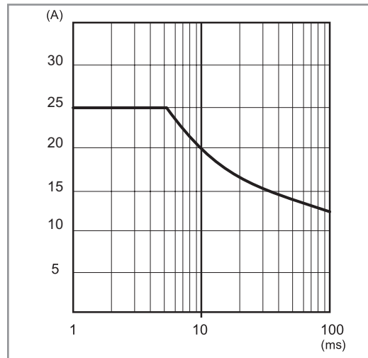
P78-10 Pico de corriente de salida en función del tiempo (78.2A)
