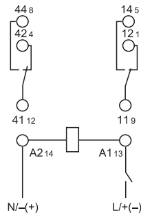
Esquema de conexión (sin señal de mando)
