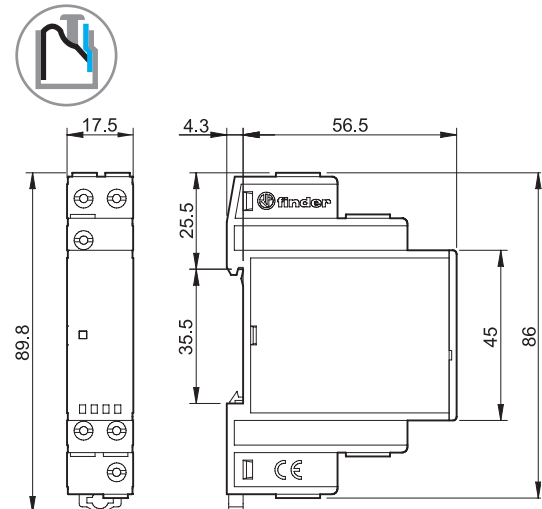
Tipo 70.61-P000 Borne push-in
