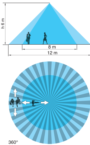
18.31...0031 - Instalaciones en techos altos
