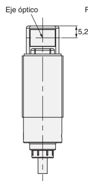
Vista posterior
