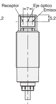
Vista posterior
