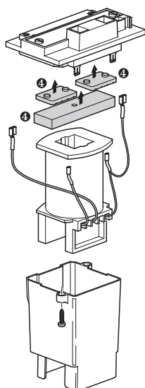
Grupo bobina completo
