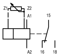
Обозначение соединений в соответствии с EN 50042
