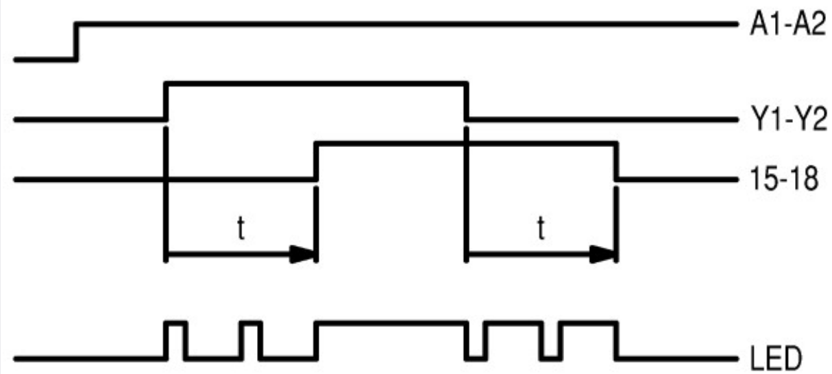
21 импульс задержки включения
