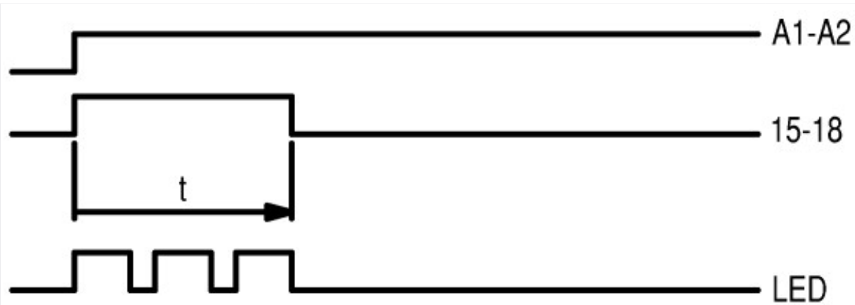
22 импульс задержки выключения
