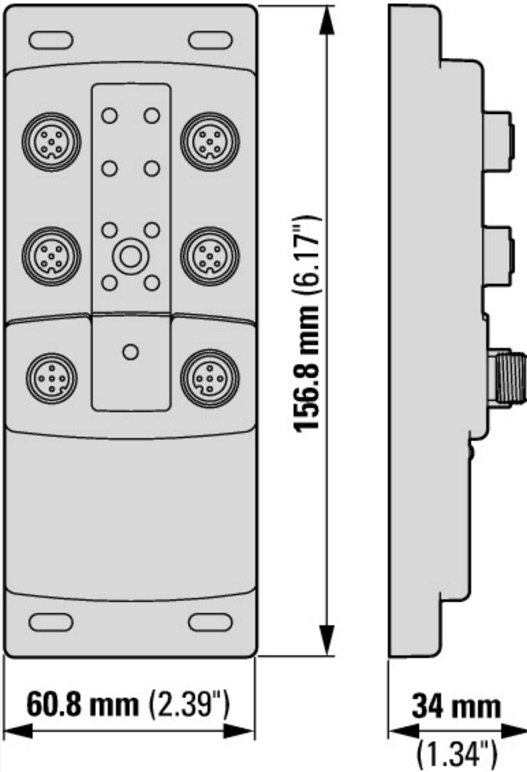
SmartWire-DT I/O modules, EU6E-SWD-... block module
