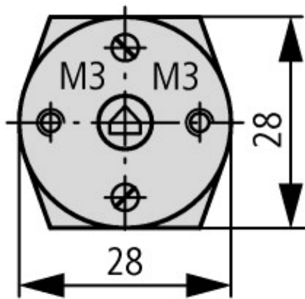
Door drilling dimensions
