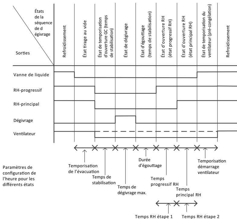
Fig. 2 - Dégivrage électrique-eau-saumure
