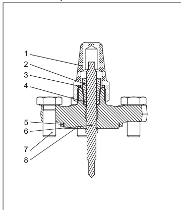
Módulo de apertura manual ICFO SS 20
