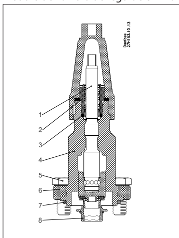
Módulo de válvula de expansión electrónica ICFA SS 20
