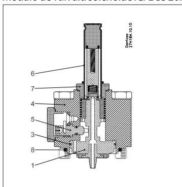
Módulo de apertura manual ICFO SS 20
