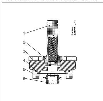
Módulo de válvula solenoide ICFE SS 20H
