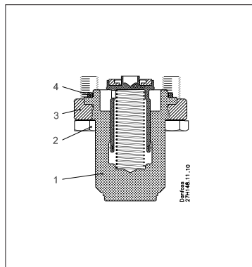
Módulo de válvula de retención ICFC SS 20
