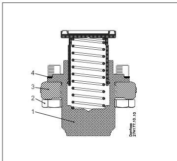
Módulo de válvula de retención ICFC SS 25
