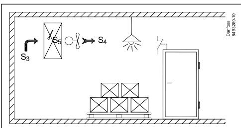
Bild 14: Kühlraumkonfiguration mit Tür-, Licht- und Heizfunktion
