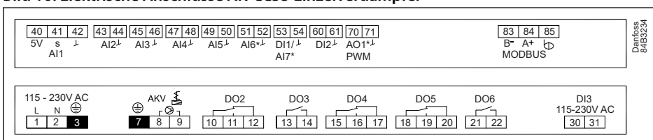
Bild 16: Elektrische Anschlüsse AK-CC55 Einzelverdampfer
