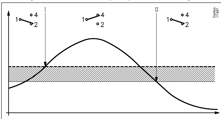
Мал 2: Функціонал контактів, при перевищенню тиску.
