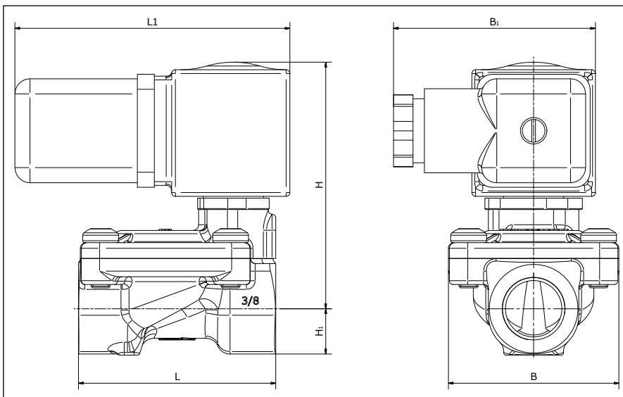
Bild 6: Maße
