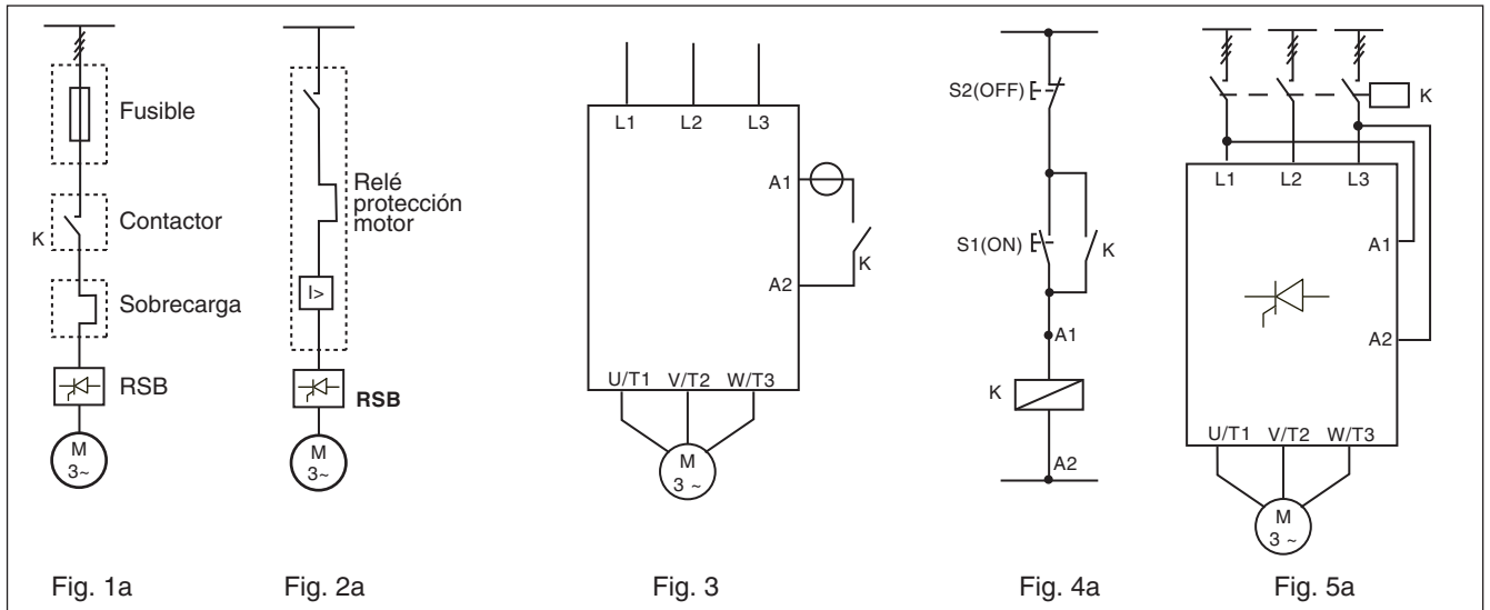
Figura 3: Control mediante interruptor de 2 posiciones
