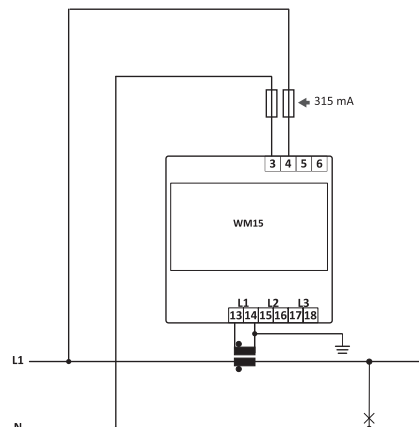
Fig. 9 Monofase (2 fili)
