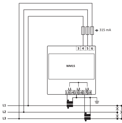
Fig. 11 Trifase senza neutro (3 fili) - ARON
