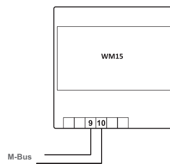
Fig. 16 M-Bus
