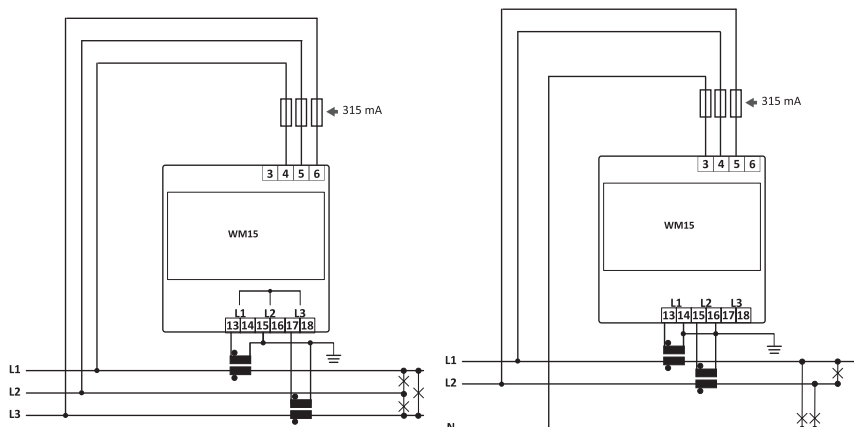
Fig. 7 Trifase senza neutro (3 fili)
