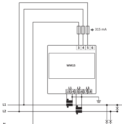
Fig. 8 Sistema bifase con neutro (3 fili)
