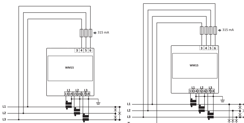
Fig. 5 Trifase senza neutro (3 fili)
