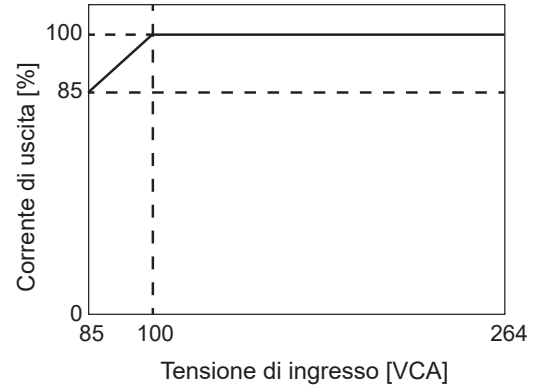
Curva di declassamento vs tensione di ingresso
