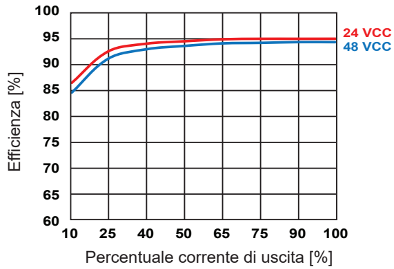
Efficienza vs al carico di uscita (230 VCA)
