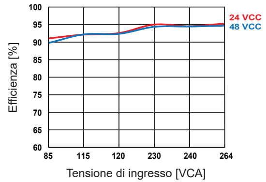
Efficienza vs le tensione di ingresso (pieno carico)
