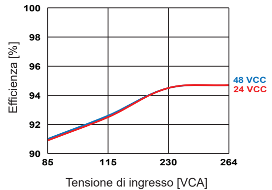
Efficienza vs le tensione di ingresso (pieno carico)
