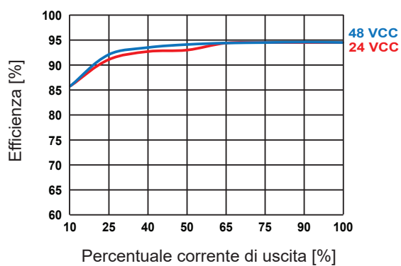
Efficienza vs al carico di uscita (230 VCA)
