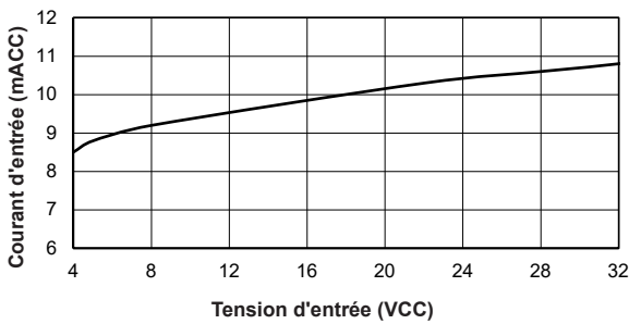
RL..D..: Courant d'entrée CC vs. tension d'entrée
