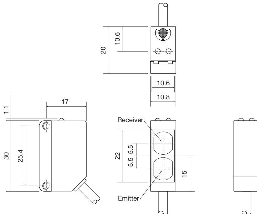
Fig. 6 Cable
