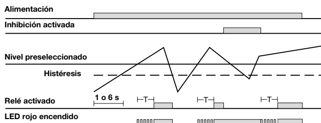
Intensidad por encima del nivel seleccionado - Función de inhibición Relé normalmente desactivado
