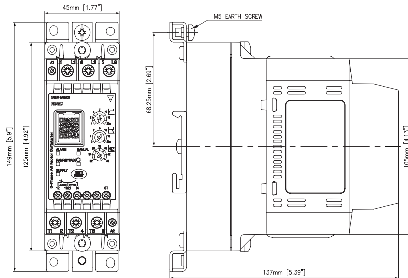
Fig. 2 RSGD4045..VX200, RSGD..25VX210 bis RSGD..45..VX210
