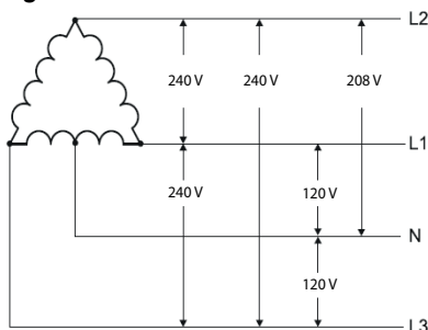
Fig. 4 Zweiphasensystem mit Nulleiter (3-drahtig)
