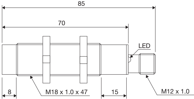
Abb. 9 Stecker CA18CAN...M1IO
