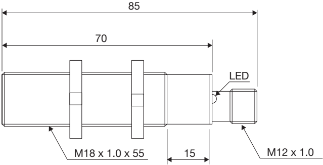
Abb. 8 Stecker CA18CAF...M1IO
