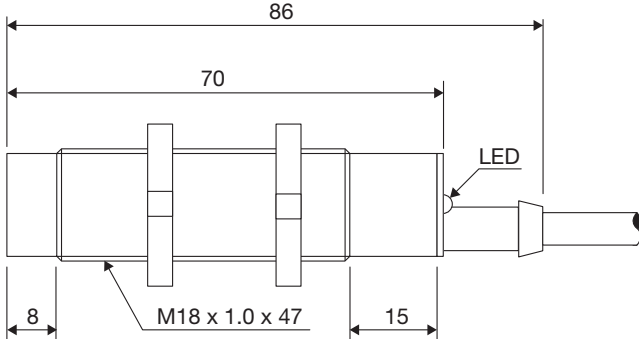
Abb. 7 Kabel CA18CAN...A2IO
