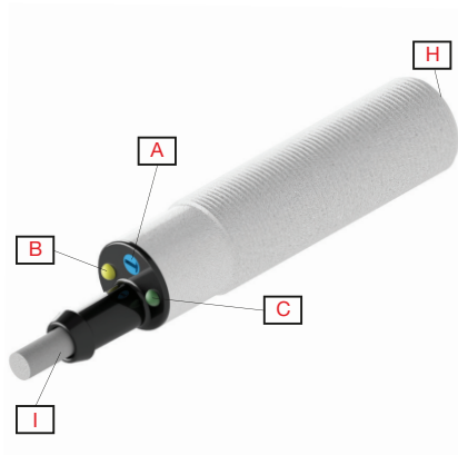
Abb. 1 CA18 Kabel
