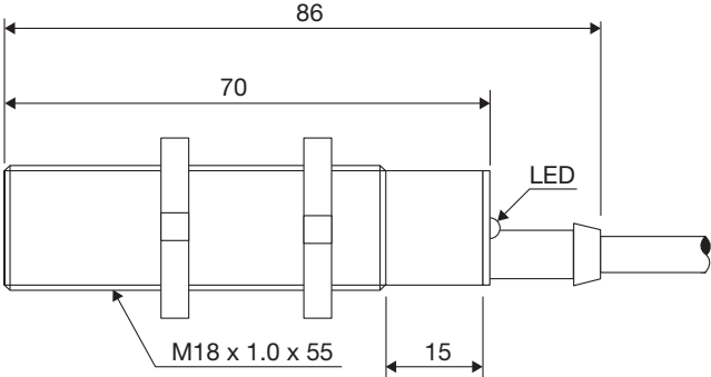
Abb. 6 Kabel CA18CAF...A2IO
