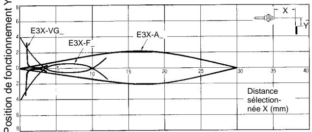
E32-D12F
