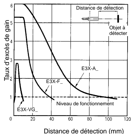
E32-D12F
