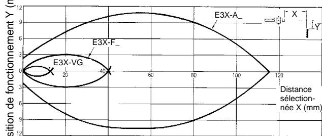
E32-D11L
