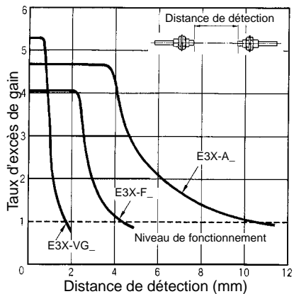
E32-T17L
