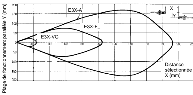
E32-T21L, E32-T22L
