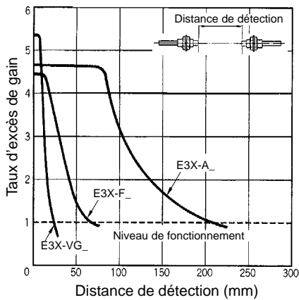
E32-T12F
