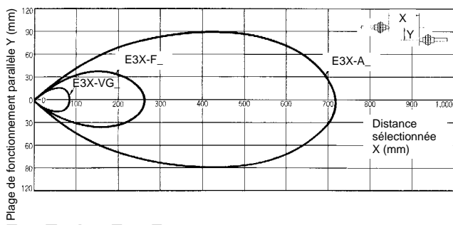
E32-T11L, +E39-F2
