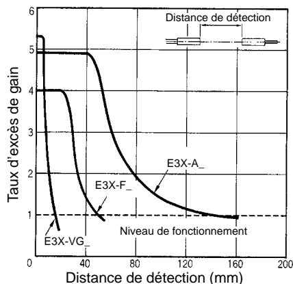
E32-T12F
