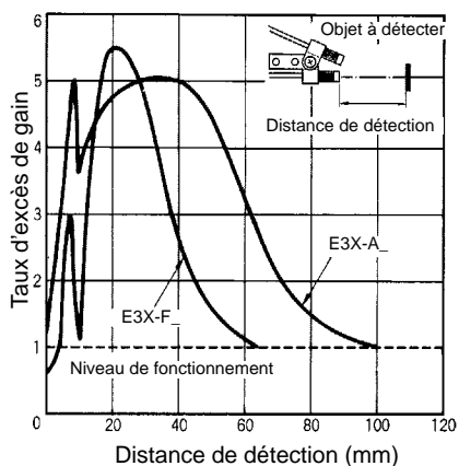
E32-T17L
