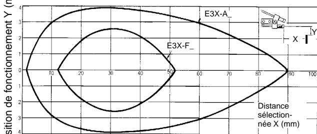
E32-T11L + E39-F3
