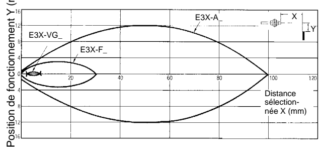
E32-D12F
