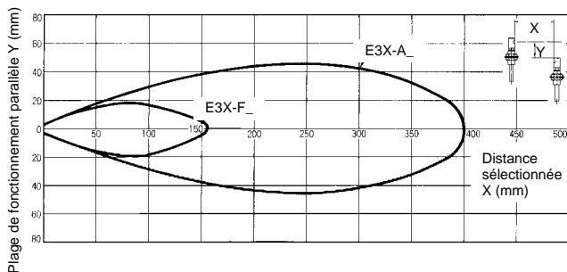
E32-T14L
