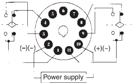
H3CR-F/-FN
