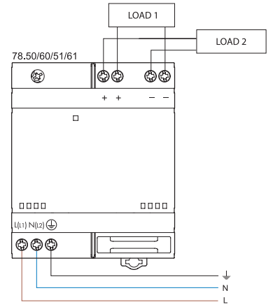
Conexiones básicas
