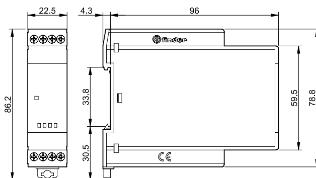
75.36 Borne de jaula
