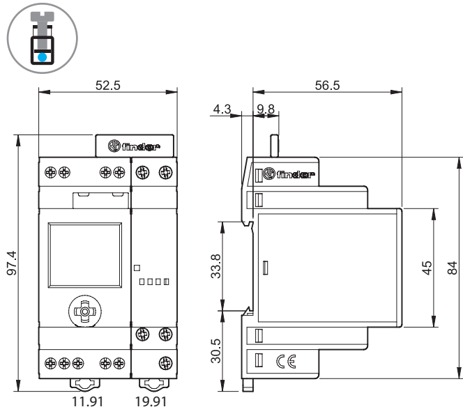
11.91 + 19.91 módulo de potencia Borne de jaula
