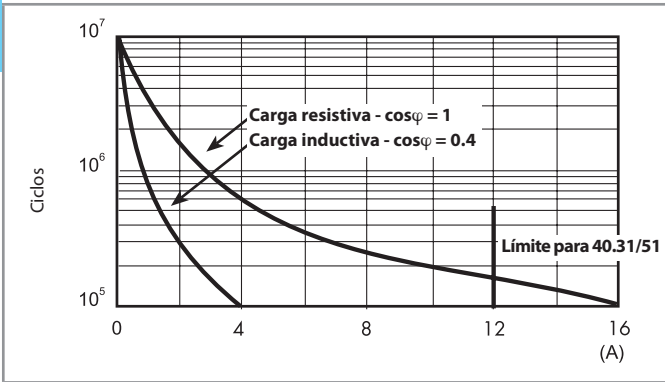
F 40.3 - Vida útil eléctrica (AC) en función de la carga
