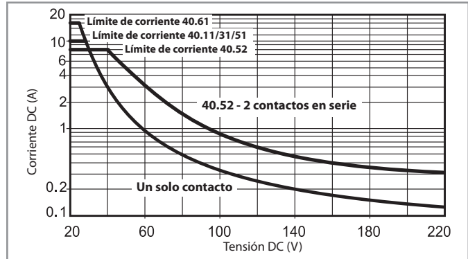
H 40.2 - Máximo poder de corte con cargas en DC1
