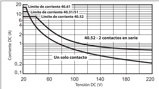
H 40.1 - Máximo poder de corte con cargas en DC1
