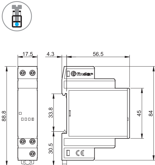
19.91 (módulo de potencia para 11.91) Borne de jaula
