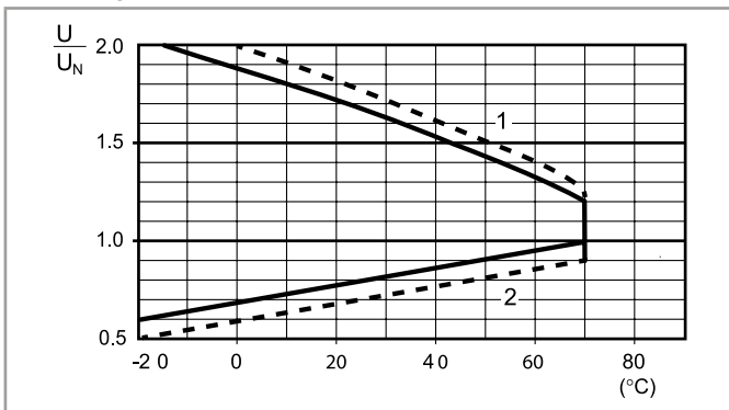
R 7S - Campo de funcionamiento de la bobina DC en función de la temperatura ambiente - 7S.12/32 / 7S.23 / 7S.14/34 / 7S.16/36
