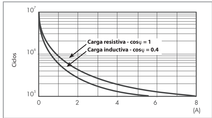
F 40.4 - Vida útil eléctrica (AC) en función de la carga
