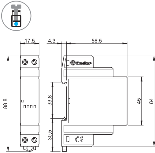
78.36 Borne de jaula
