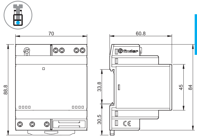
78.1B Borne de jaula
