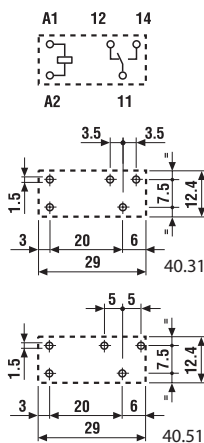
Vista parte inferior Largo de terminal 5.3 mm para CI o zócalo
