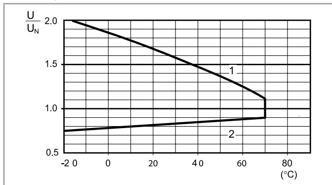
R 7S - Campo de funcionamiento de la bobina AC en función de la temperatura ambiente - 7S.12/32 / 7S.23 / 7S.14/34 / 7S.16/36
