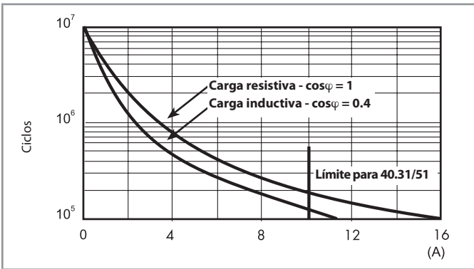
F 40.5 - Vida útil eléctrica (AC) en función de la carga
