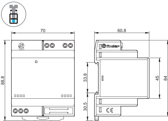
78.51 / 78.61 Borne de jaula
