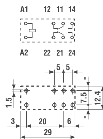
Vista parte inferior Largo de terminal 5.3 mm para CI o zócalo
