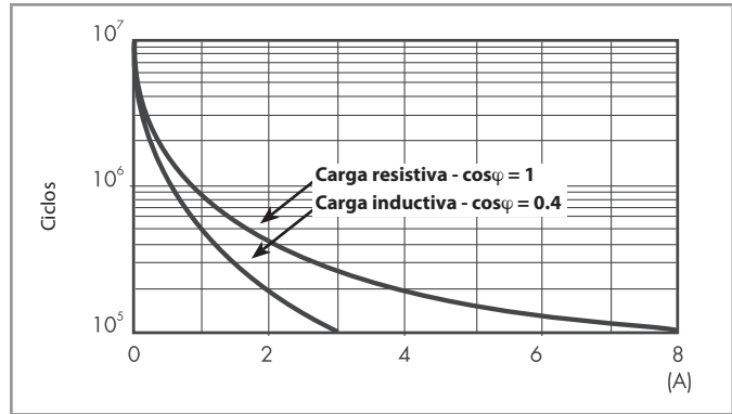
F 40.4 - Vida útil eléctrica (AC) en función de la carga
