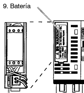
Lateral derecho (CPU con salidas a relé)
