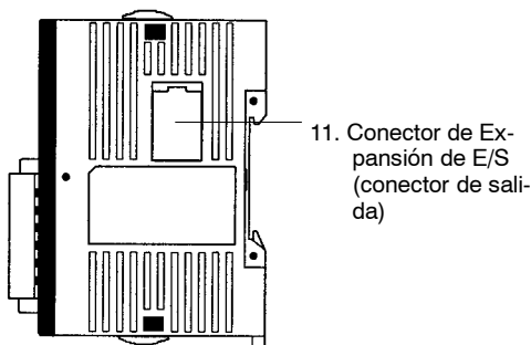
Lateral derecho (CPU con salidas a relé)
