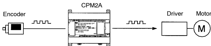
Pulsos emitidos a frecuencia múltiplo de la frecuencia de entrada
