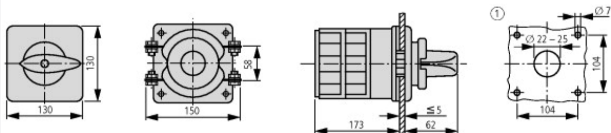
① Drilling dimensions door
