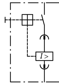
M...-PKZ2(4)
