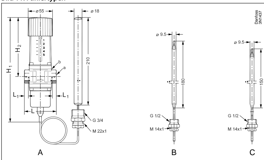
Bild 11: Fühlertypen
