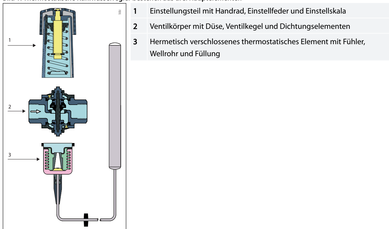
Bild 1: Thermostatische Kühlwasserregler bestehen aus drei Hauptelementen
