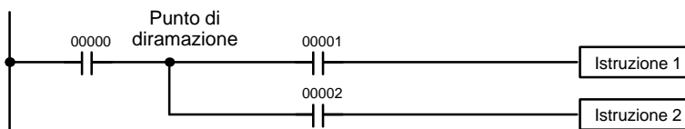
Circuito B (codifica errata)
