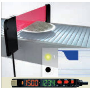
Les deux sortie du E3X-DA-S peuvent être utilisées pour détecter deux niveaux de luminosité différents
