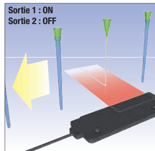
En combinaison avec la fonction de double sortie de l'amplificateur E3X-DA-S, les fibres de surveillance de zone à réflexion directe peuvent détecter de très petits objets (tels que des aiguilles) ainsi qu'un deuxième état (présence du couvercle, par exemple). Le faisceau de zone compense les variations de position aux vitesses élevées.
